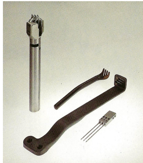
Pezzi che compongono la testina a 3 aghi Parts forming the 3-needle post Piezas que componen el poste de 3 agujas
